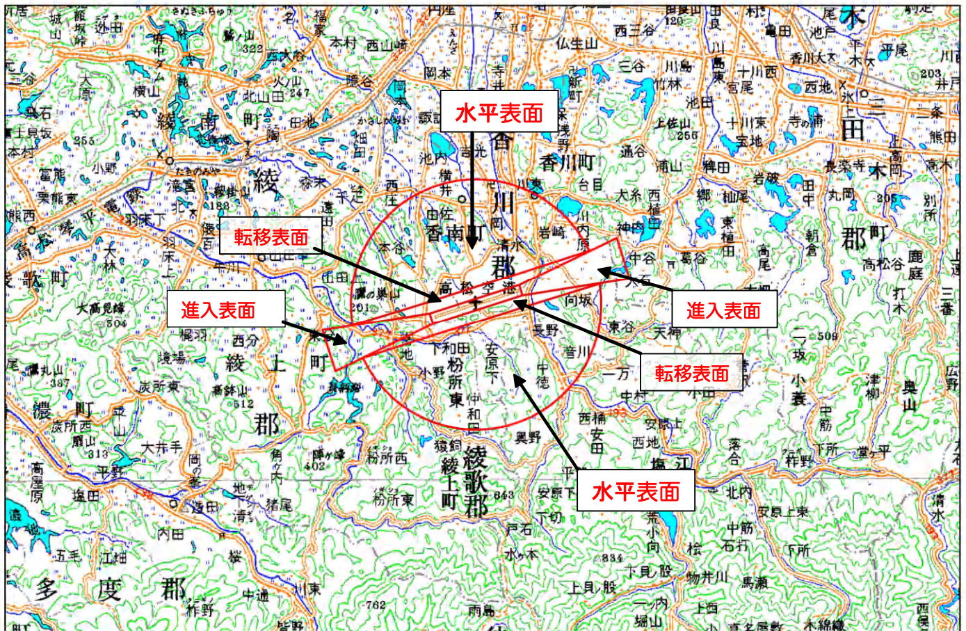
高松空港の制限表面区域図
